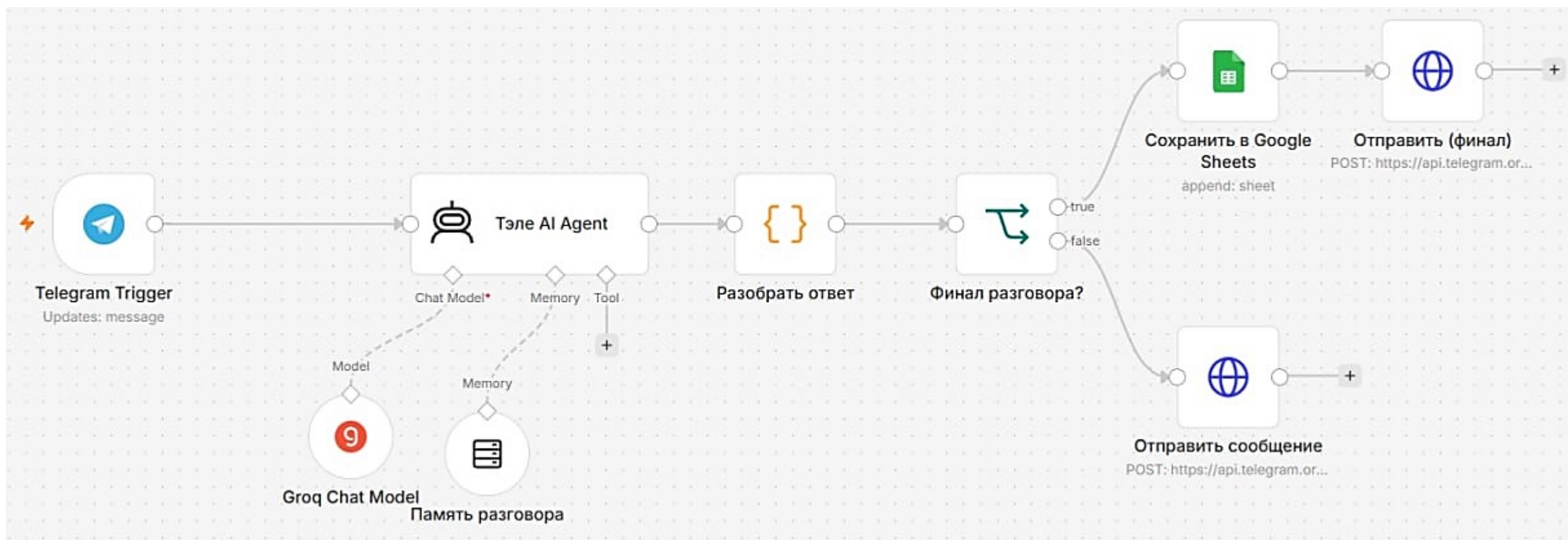
Рис. Workflow из n8n
